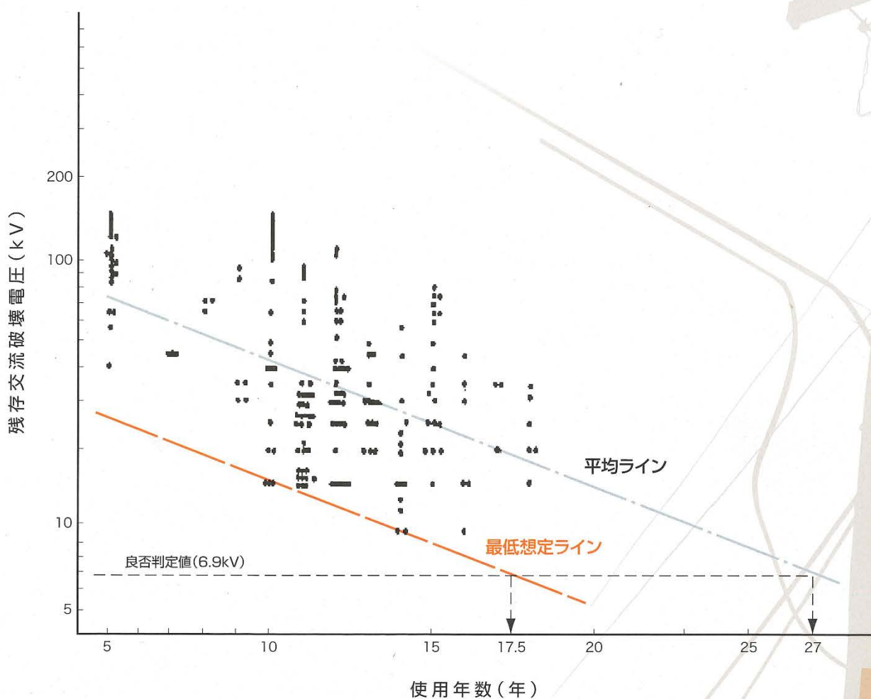
【高圧CVケーブルの長期性能評価】高圧CVケーブルの保守・点検指針 技資第116号Dより
